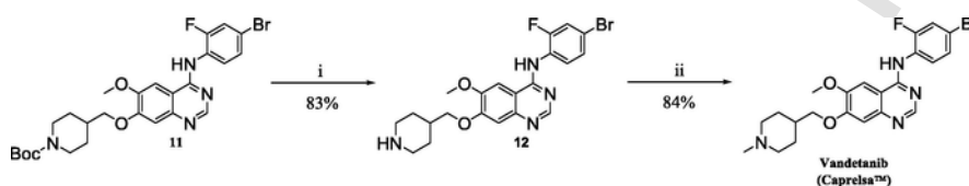
Scheme 5. i) TFA, DCM, rt, 2 h; ii) HCHO, AcOH, NaBH(OAc) 3 , MeOH, DCM, rt, 2 h.
